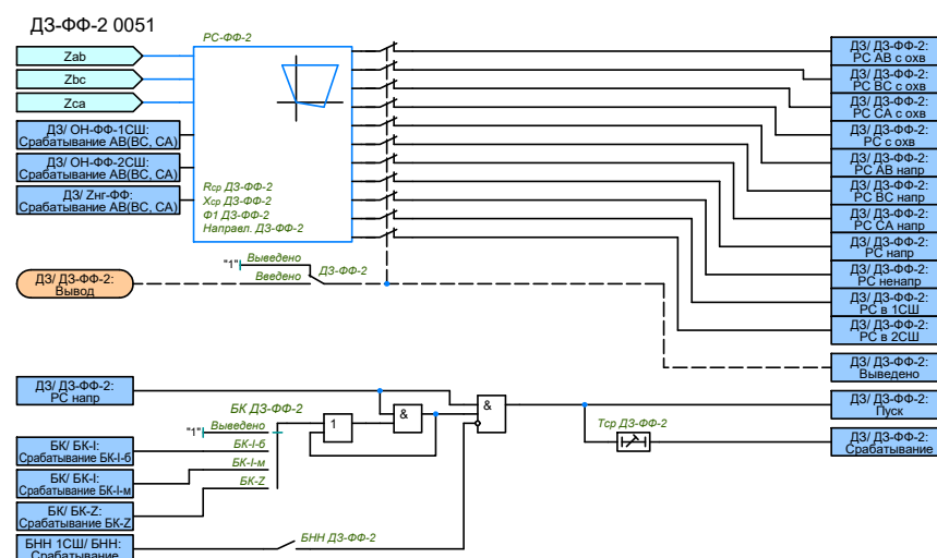
Рисунок 2.11 – Функциональная схема ДЗ-ФФ-2(4)
