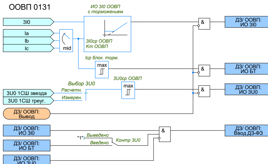
Рисунок 2.9 – Функциональная схема ООВП
