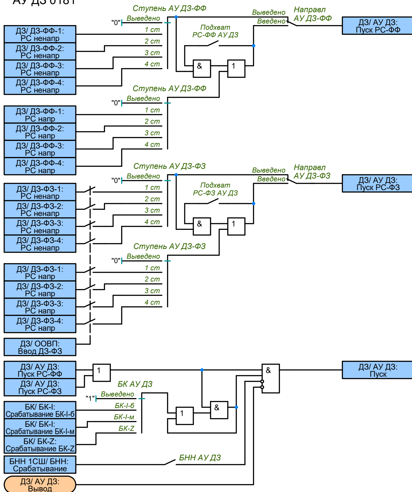
Рисунок 2.16 – Функциональная схема пуска АУ ДЗ
