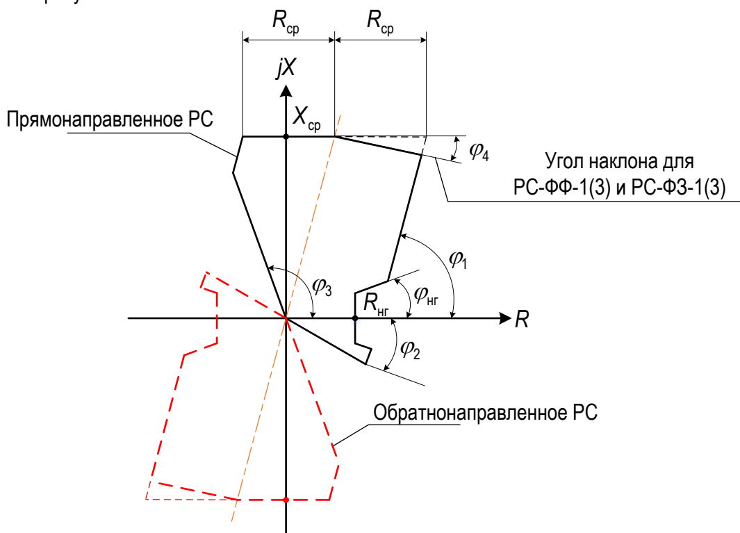
Рисунок 2.6 – Характеристики срабатывания направленного РС
