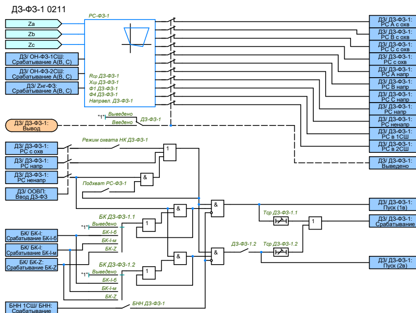
Рисунок 2.12 – Функциональная схема ДЗ-ФЗ-1(3)
