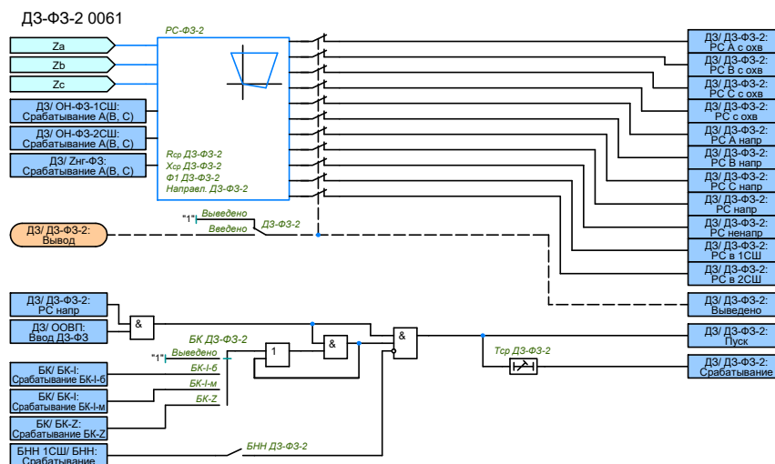
Рисунок 2.13 – Функциональная схема ДЗ-Φ3-2(4)
