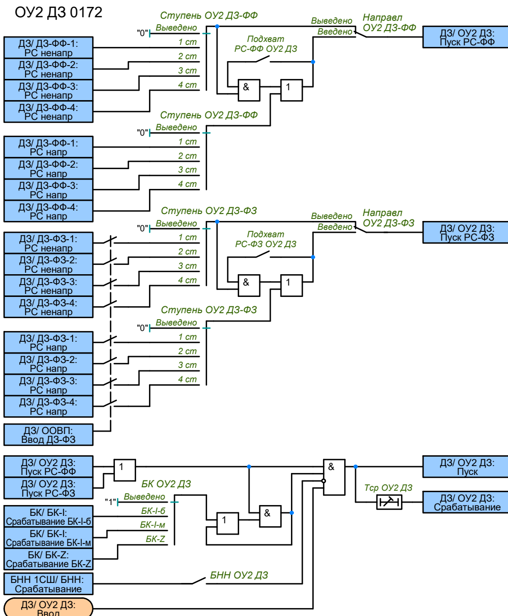
Рисунок 2.14 – Функциональная схема ОУ2 ДЗ
