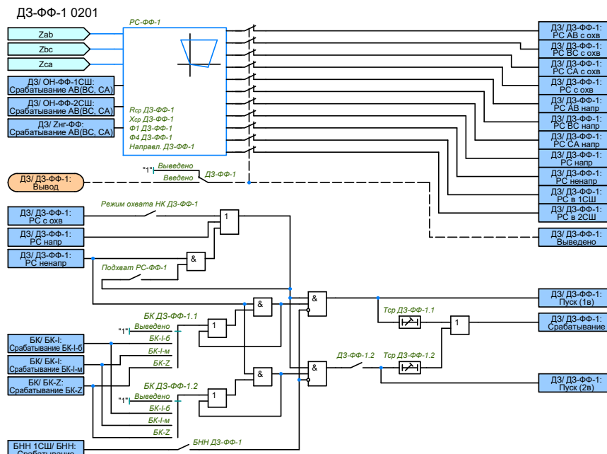
Рисунок 2.10 – Функциональная схема ДЗ-ФФ-1(3)
