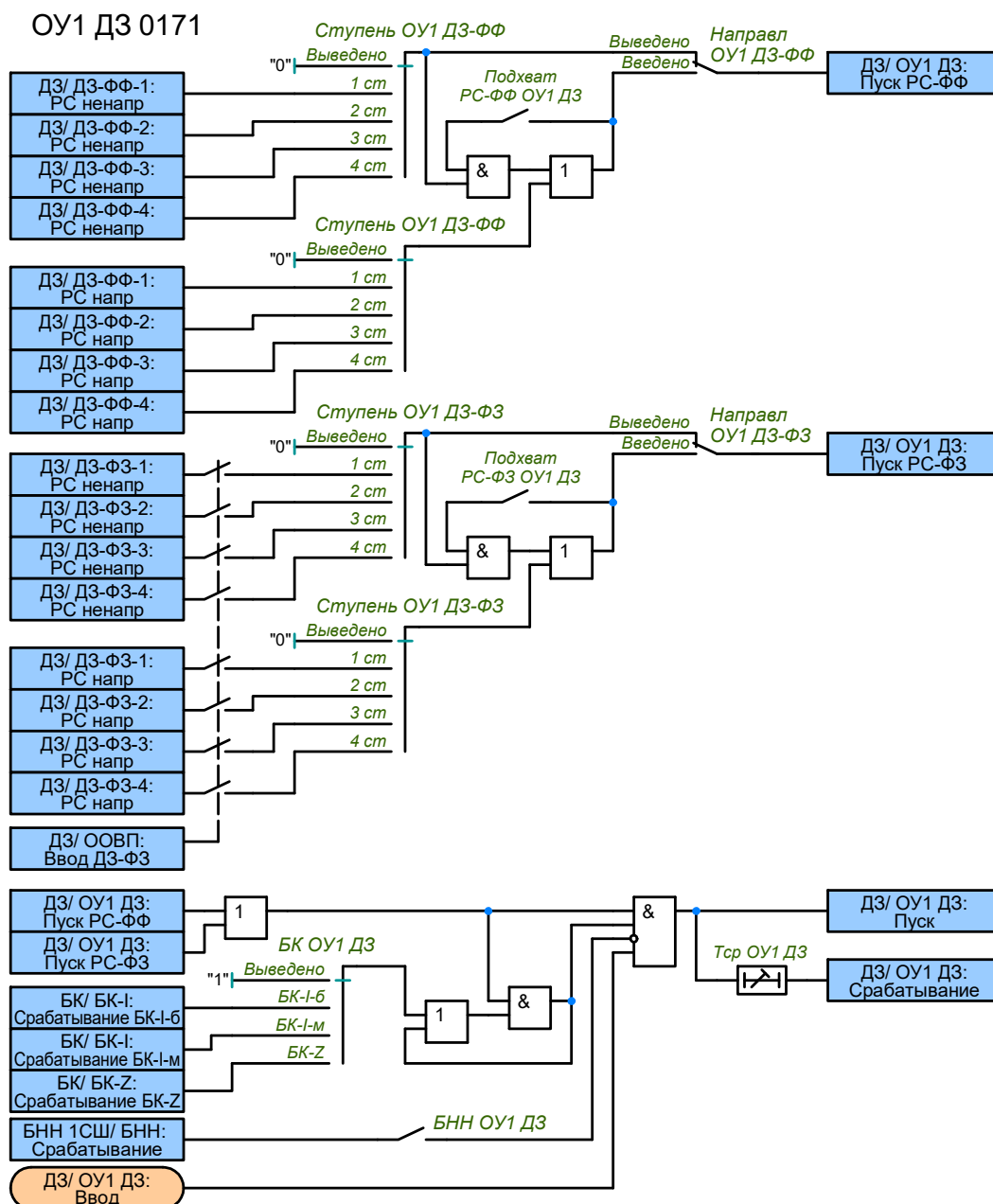
Рисунок 2.15 – Функциональная схема ОУ1 ДЗ
